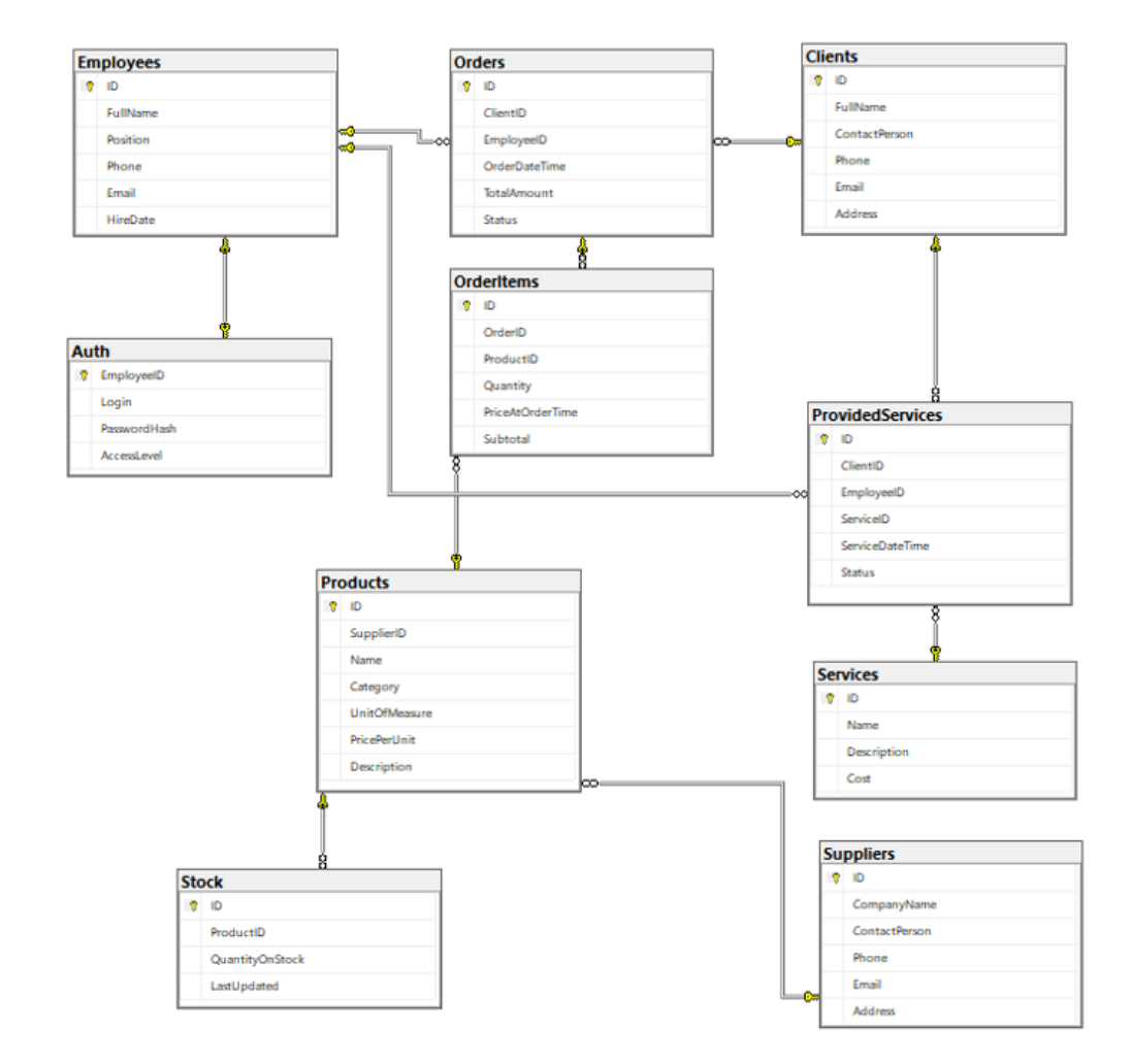
Рисунок 3.25. Физическая ER диаграмма
